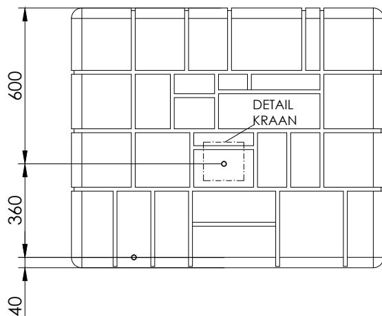
VOORAANZICHT
