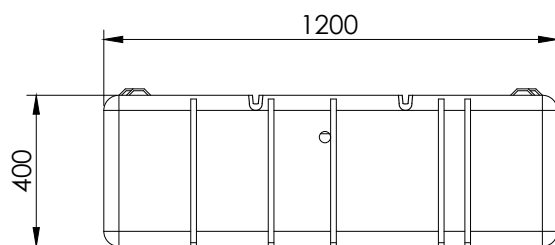
BOVENAANZICHT
