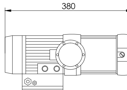
VOORAANZICHT
