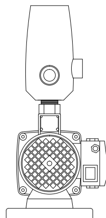
LINKERZIJAANZICHT
